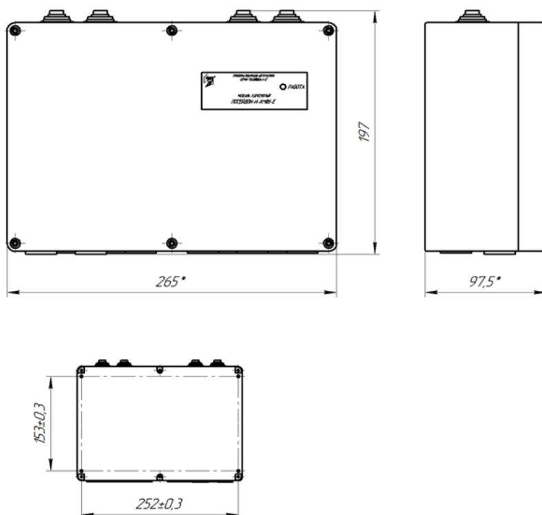
Рисунок 1 - Внешний вид прибора, в настенном исполнении
