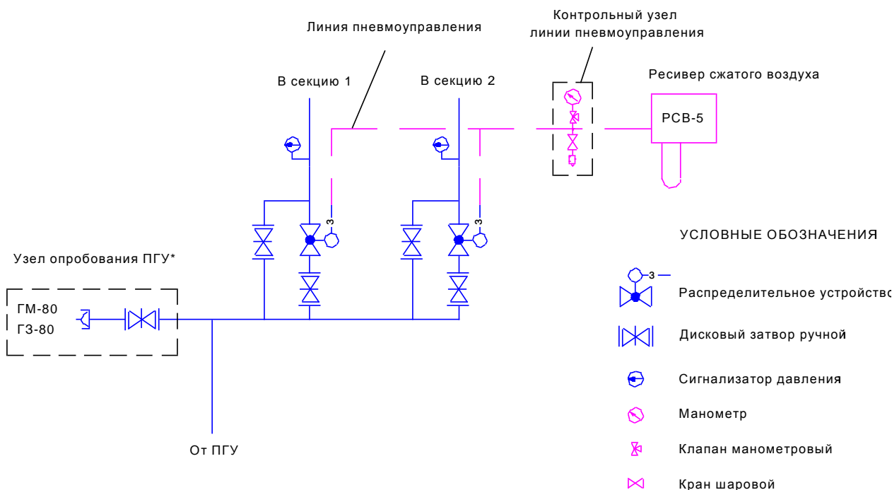
Рисунок 5.13 Пример построения узла управления
