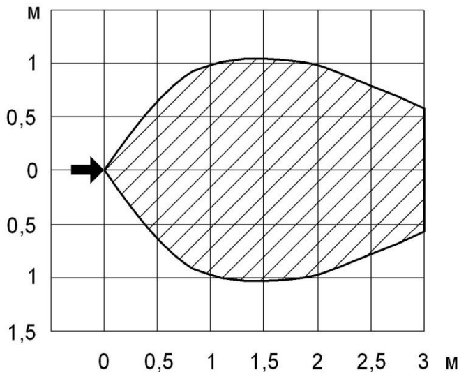
Рисунок 3.7 Карта орошения ОПР-375П при горизонтальной установке на высоте 0,6 м
