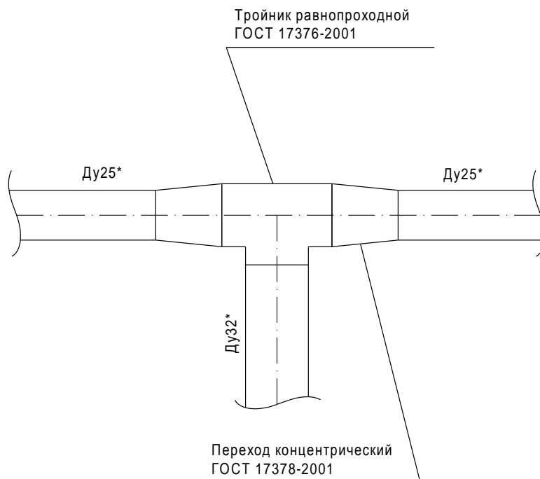
Рисунок 5.6 Соединение трубопроводов при разветвлении на трубы меньшего диаметра
