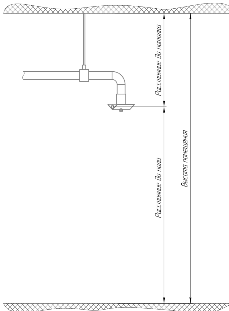
Рисунок 3.3 Схема расположения оросителя ОПР-375Н на распределительном трубопроводе
