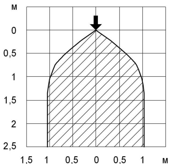
Рисунок 3.6 Карта орошения ОПР-375П при вертикальной установке на высоте 2,5 м
