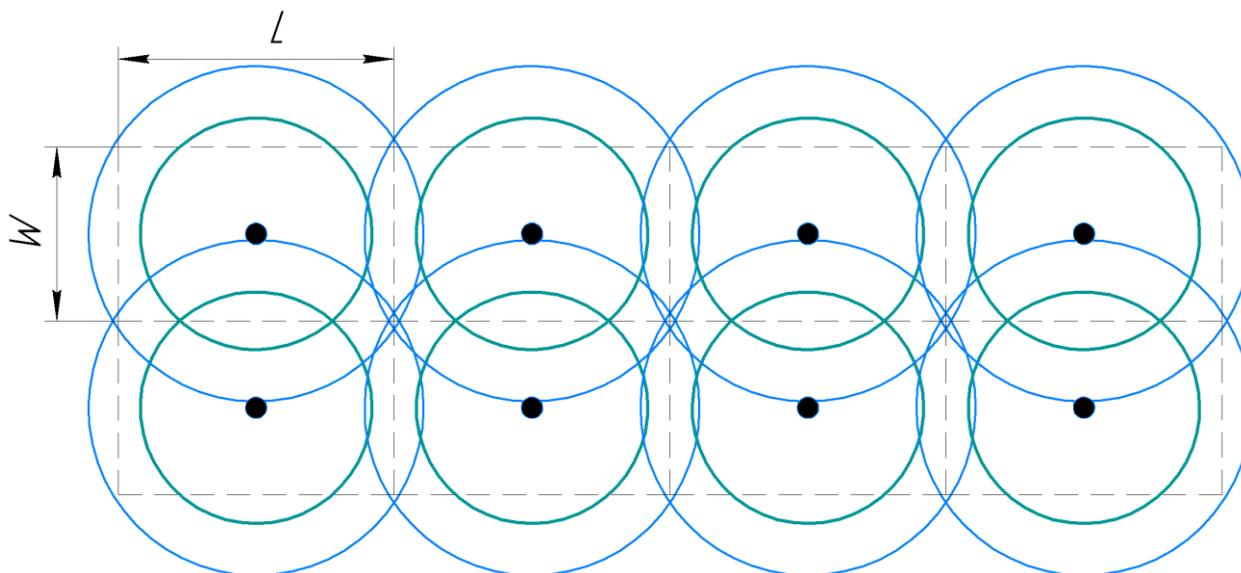
Рисунок 3.5 Схема расположения оросителей ОПР-375Н по площади
