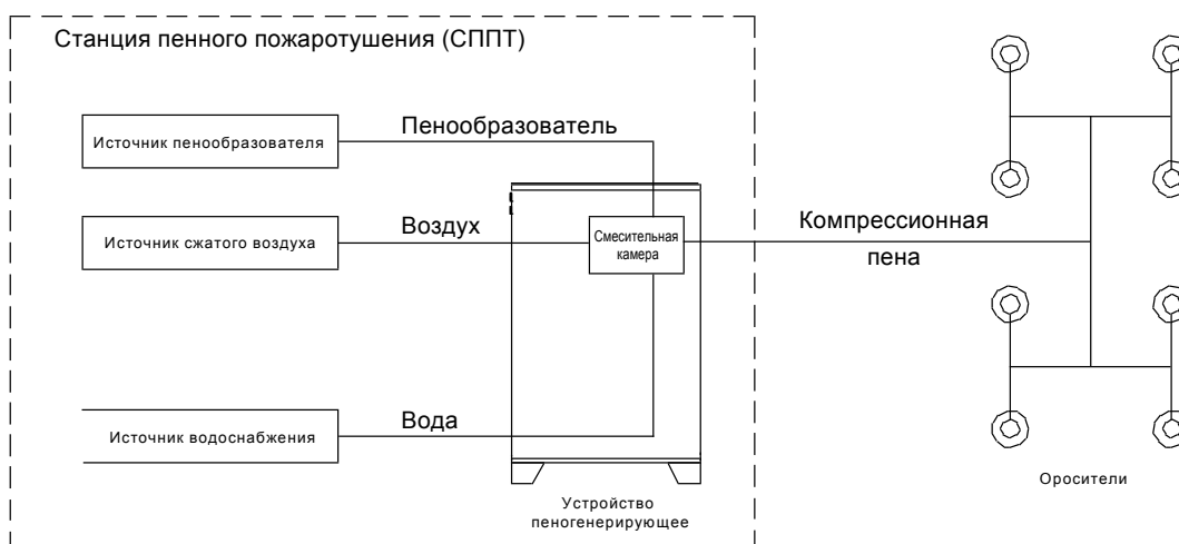
Рисунок 3.1 Общая схема установки пожаротушения
