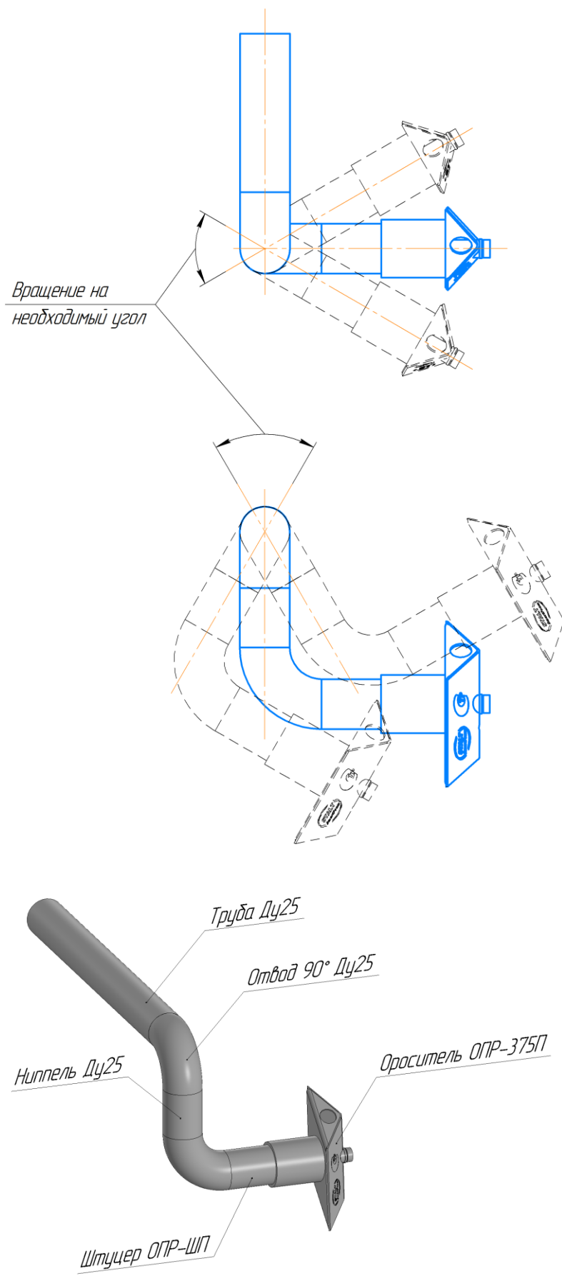
Рисунок 3.8 Рекомендуемая схема установки оросителей ОПР-375П
