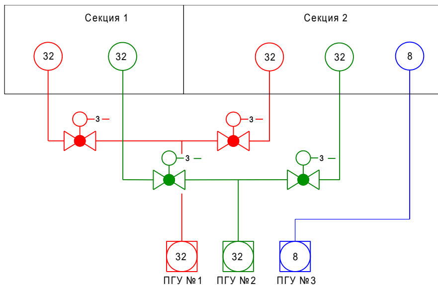
5.12 Пример комбинированной установки на две секции пожаротушения
