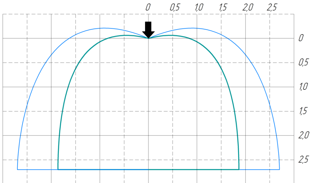
Рисунок 3.4 Зона орошения ОПР-375Н (толстой линией показана зона орошения с нормативной интенсивностью, тонкой – максимальный разлёт пены)
