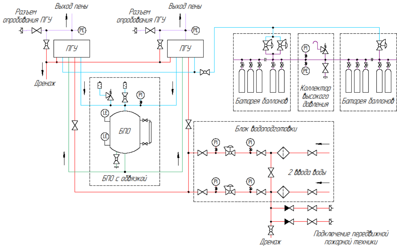
Рисунок 4.1 Схема трубопроводов станции пенного пожаротушения (пример)
